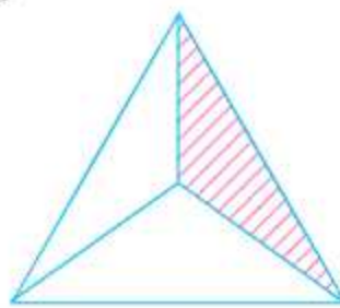
ਤਿਕੋਣਾਕਾਰ ਪਿਰਾਮਿਡ
