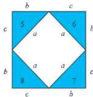
ਵਰਗ A
