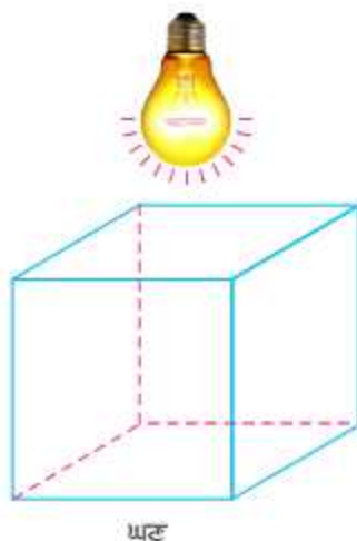
ਘਣ
