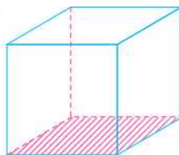
ਘਣ
