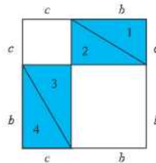
ਵਰਗ B
