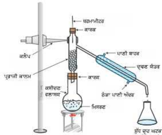
ਚਿੱਤਰ 2.10 : ਪ੍ਰਭਾਜੀ ਕਸ਼ੀਦਣ
