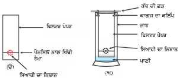
ਚਿੱਤਰ 2.8 : ਕਰੋਮੈਟੋਗਰਾਫੀ ਦੁਆਰਾ ਕਾਲੀ ਸਿਆਹੀ ਵਿੱਚ ਮੌਜੂਦ ਡਾਈਆਂ ਦਾ ਨਿਖੇੜਨ
