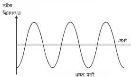
ਚਿੱਤਰ 12.10 : ਧੀਮੀ ਧੁਨੀ ਦਾ ਅਯਾਮ ਘੱਟ ਹੁੰਦਾ ਹੈ ਅਤੇ ਤੇਜ਼ ਧੁਨੀ ਦਾ ਅਯਾਮ ਜ਼ਿਆਦਾ ਹੁੰਦਾ ਹੈ।
