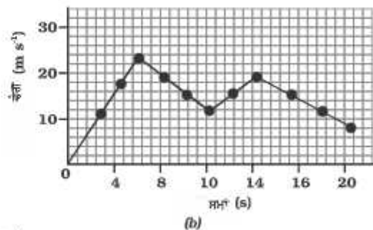
ਚਿੱਤਰ 8.7 ਅਸਮਾਨ ਪ੍ਰਵੇਗਿਤ ਗਤੀ (Non-Uniformly Accelerated Motion) ਨਾਲ ਚਲ ਰਹੀ ਕਿਸੇ ਵਸਤੂ ਦੇ
